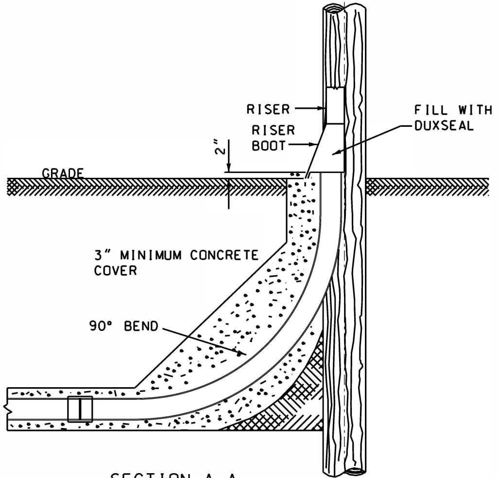
SECTION A-A
